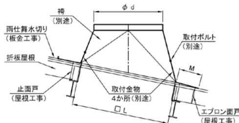
屋根設置 袴(オプション)納まり図
